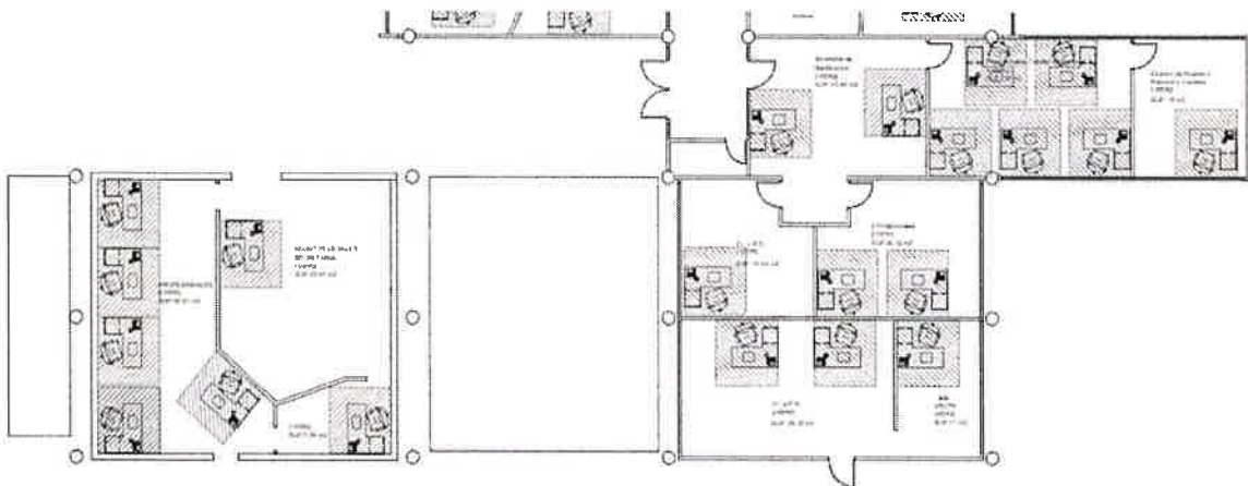
PRIMER PISO RECTORIA Y ASUNTOS LEGALES FSC/AI A- 1/100
