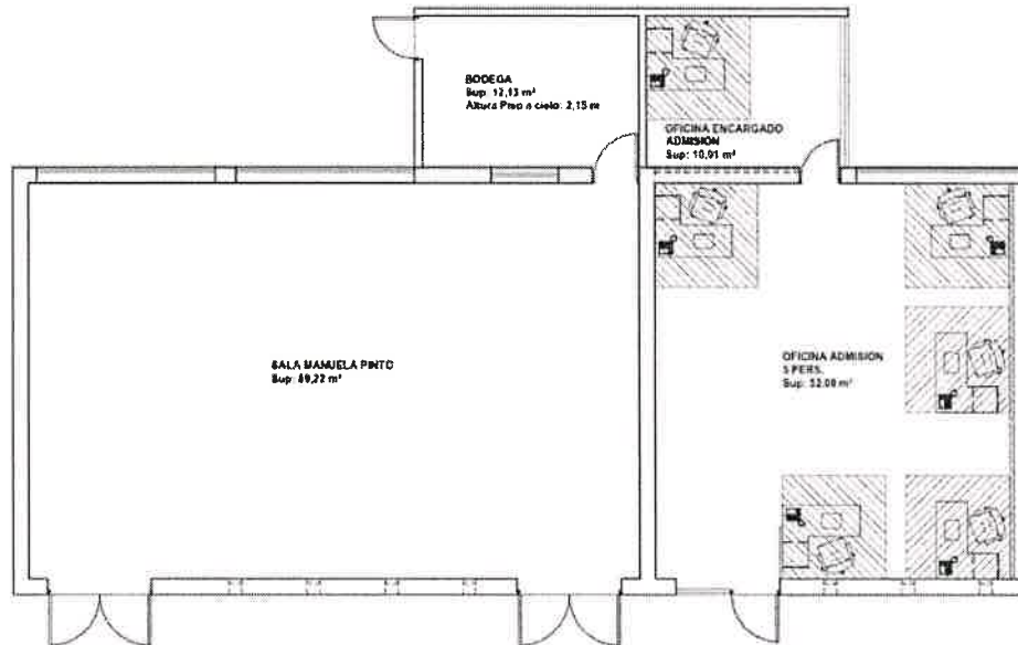
ZOCALO EDIFICIO 18 SEPT. ADMISION ESCALA: 1/100
