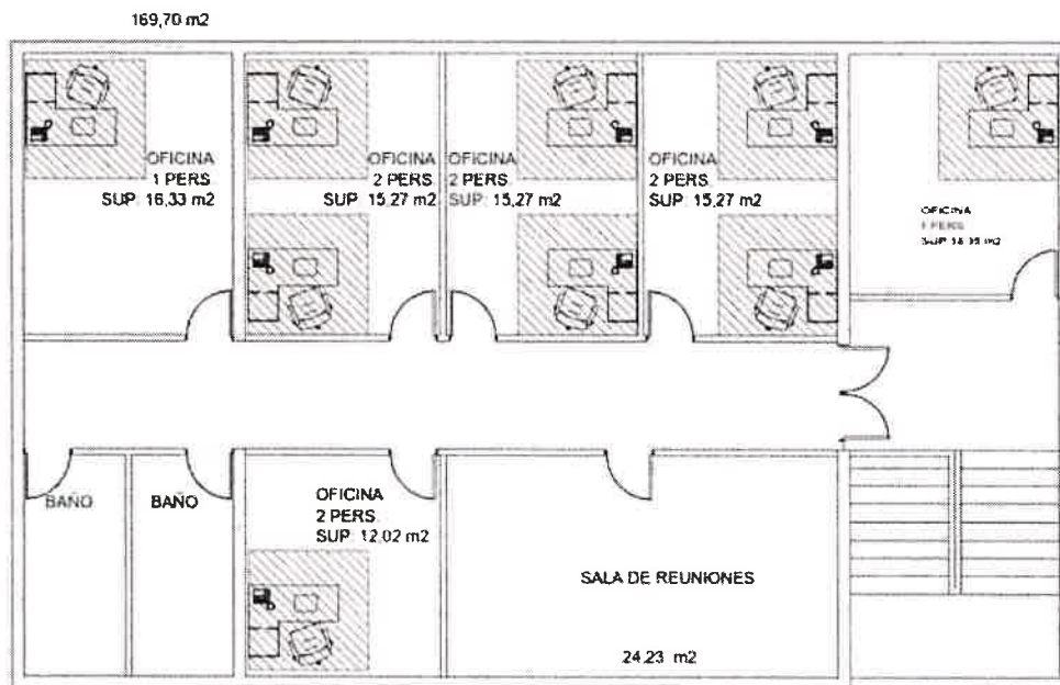
SEGUNDO PISO DOCENCIA ESCALA: 1/100
